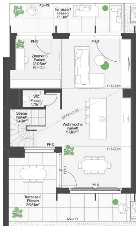
5. Obergeschoß
