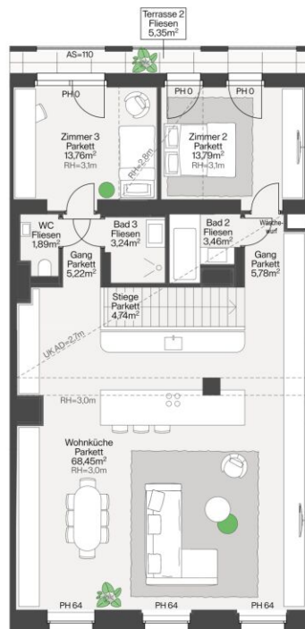
3. Obergeschoß
