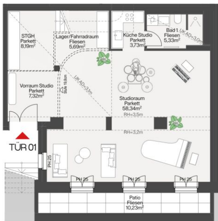
Sockelgeschoß
